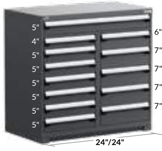
13 DRAWERS R5KHE-4413 48" x 24" x 46" R5KHG-4413 48" x 27" x 46"
