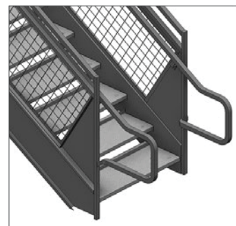
Modèle 4 2 traverses + main courante + grille de protection
